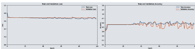
(f) CNN-SGD - DS_3
