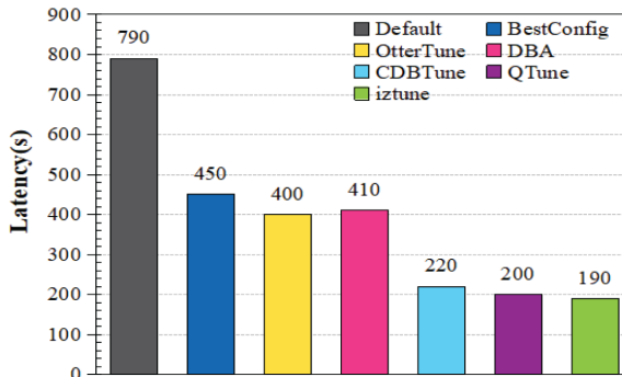
(b) TPC-H(RO)
